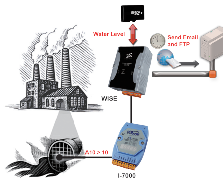
▲ Data Logger function
